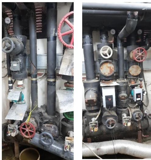
Εικόνα 2. Υφιστάμενος συλλέκτης λεβητοστασίου
